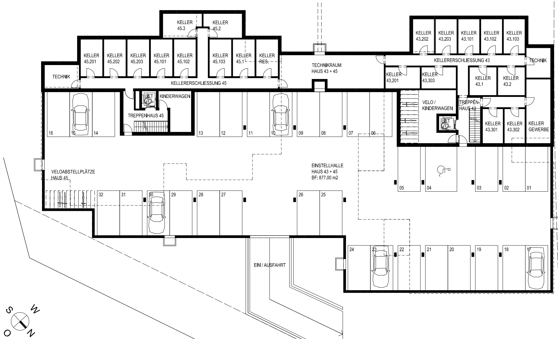
GARAGEN UNTERGESCHOSS BAHNHOFSTRASSE 43 + 45 MST. 1:250
