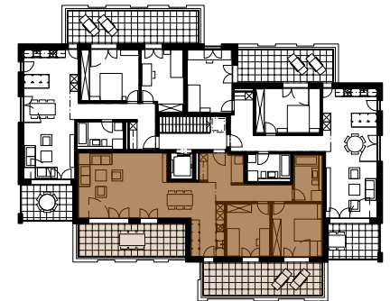
ÜBERSICHT 3.OG HAUS BAHNHOFSTRASSE 43 MST. 1:500
