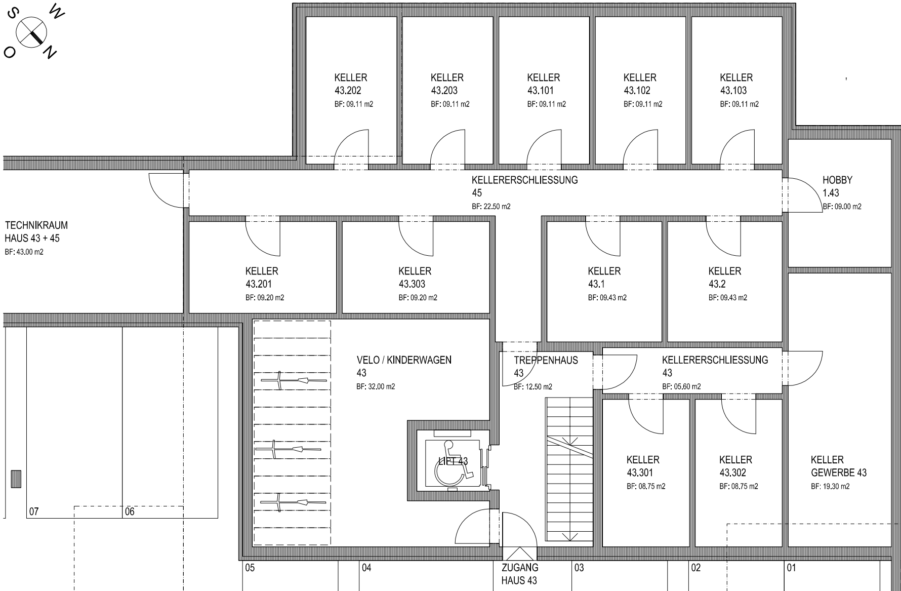
GRUNDRISS UNTERGESCHOSS HAUS 43 MST. 1:100
