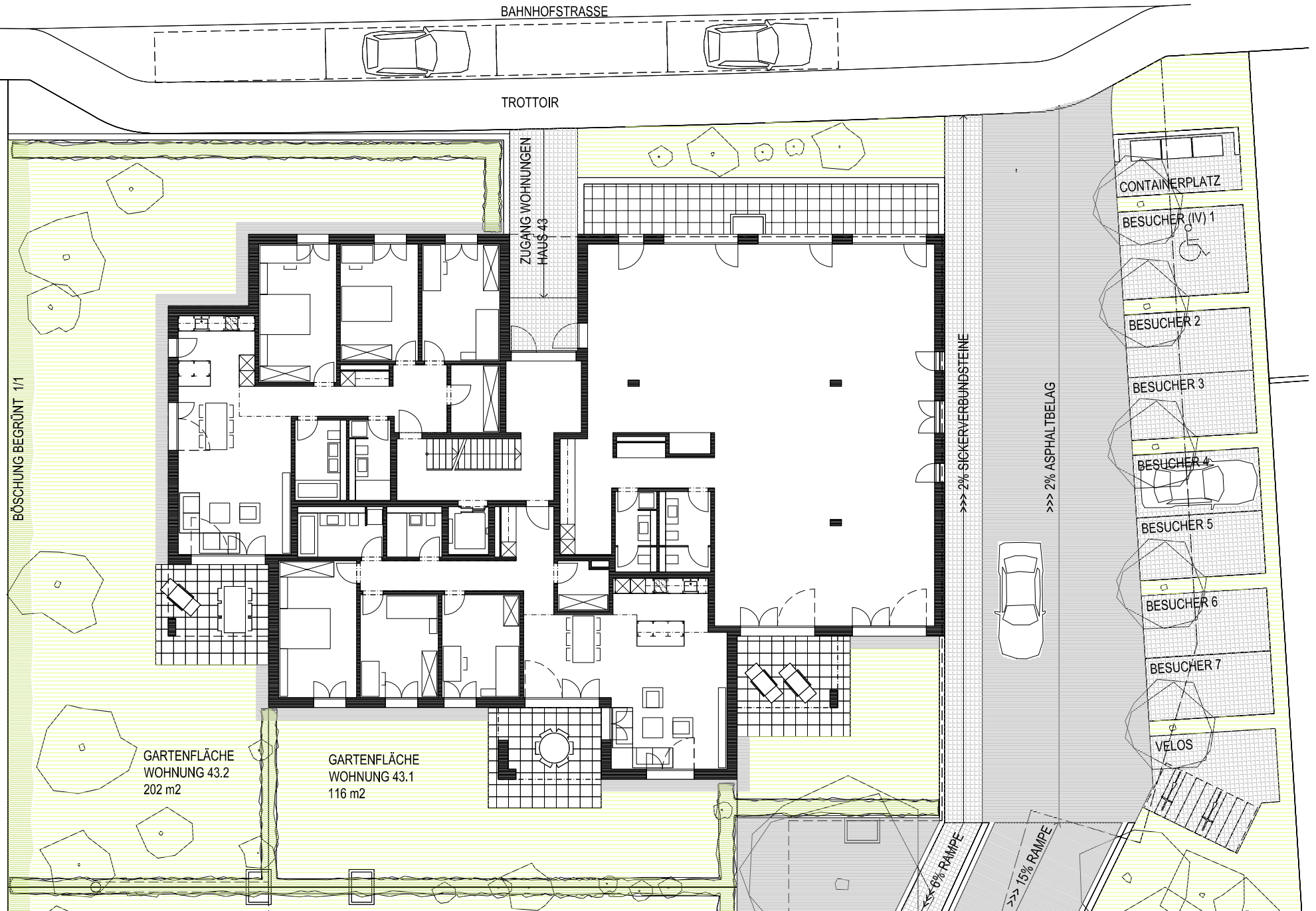
GRUNDRISS ERDGESCHOSS MIT UMGEBUNG HAUS 43 MST. 1:200
