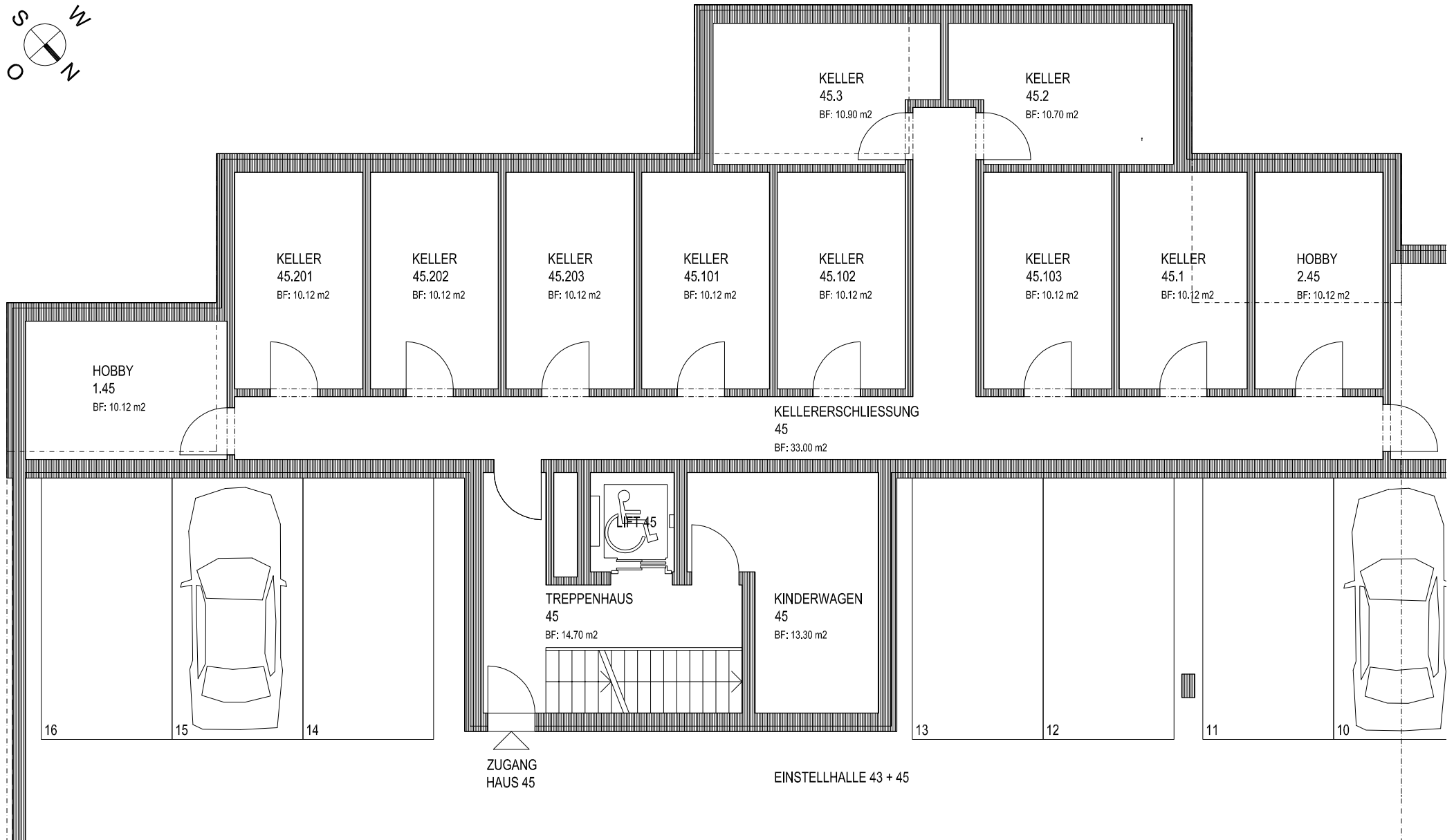
GRUNDRISS UNTERGESCHOSS HAUS 45 MST. 1:100
