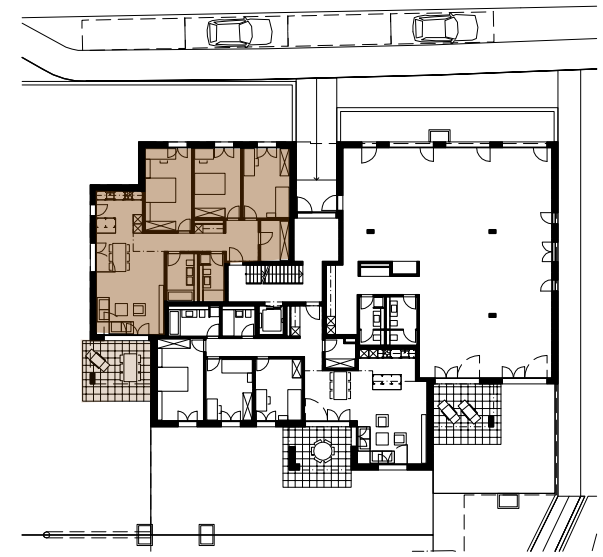
GRUNDRISS ERDGESCHOSS MST. 1:100
